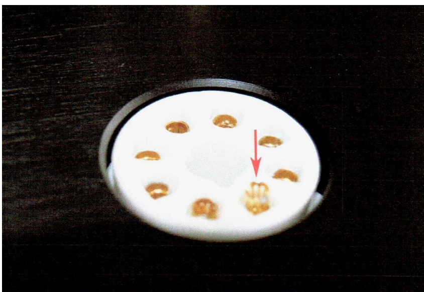
Рис. 2. Внутренняя пружина (частично вынута)
